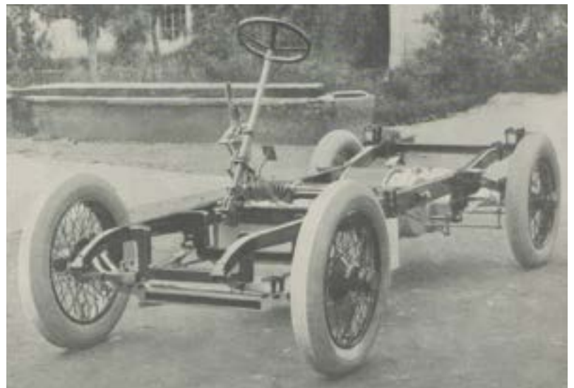
Motor, Räder und Rahmen des 12-PS-Elektromobils von Gmür mit einer Reichweite von bis zu 140 km.
